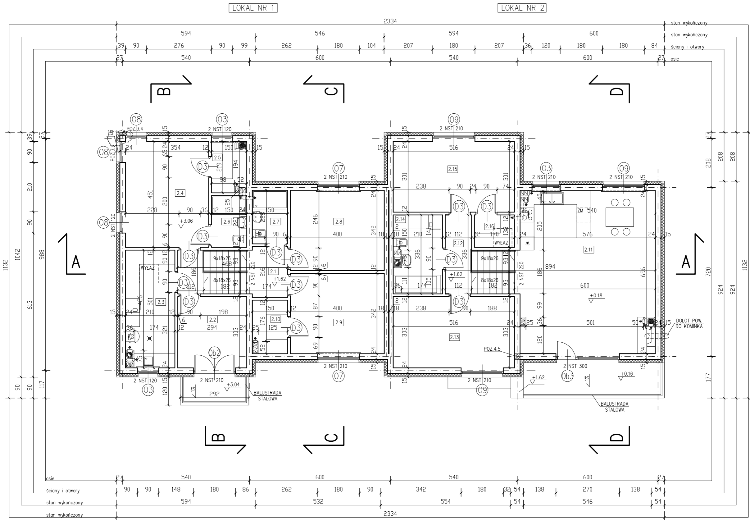
RZUT PIĘTRA 1:100
