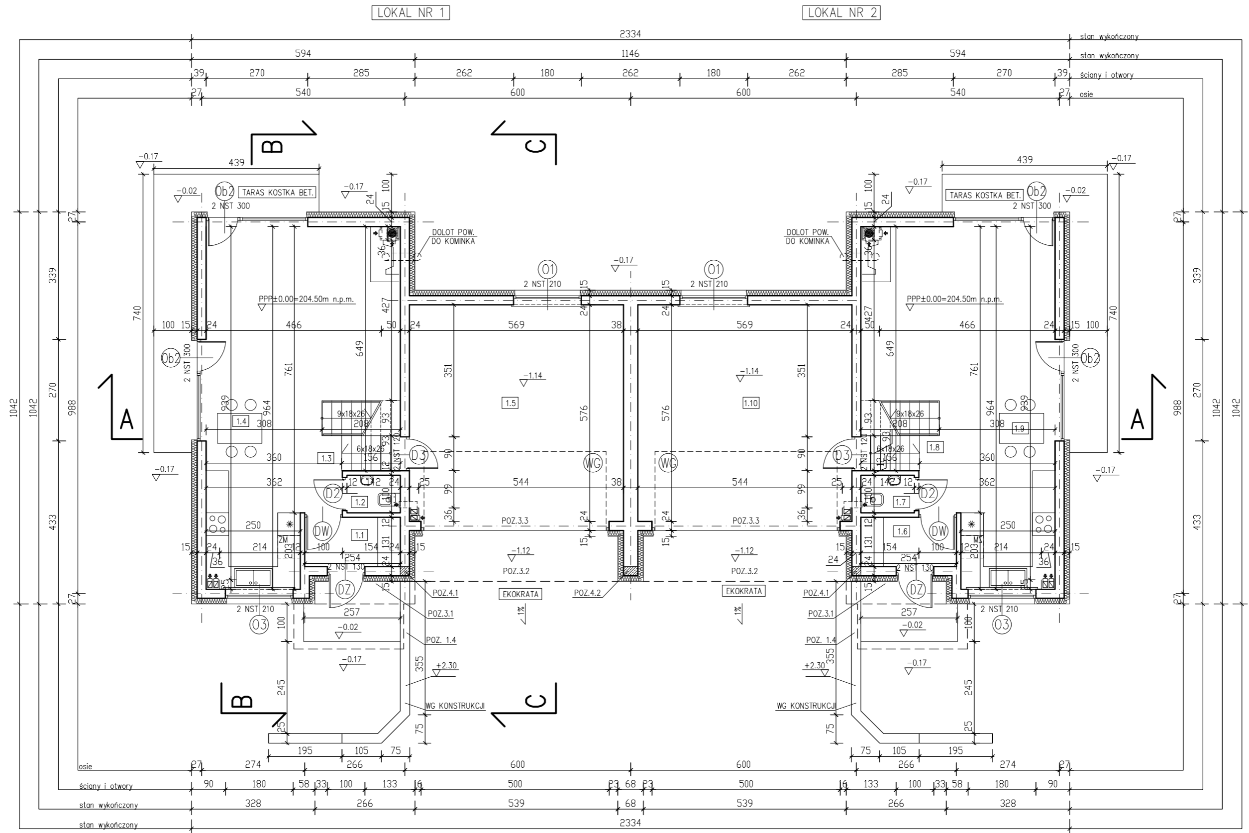
RZUT PARTERU 1:100
